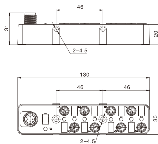
IO-Link输入输出模块-M8
