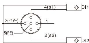
NPN型双输入
