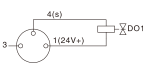
NPN型输出
