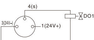
PNP型输出
