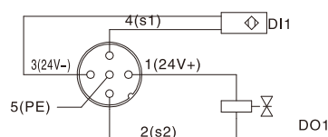
NPN型输入和输出
