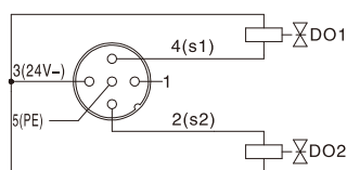
PNP型双输出
