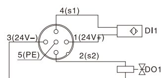
PNP型输入和输出
