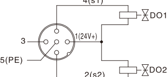
NPN型双输出
