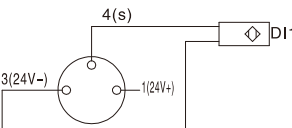
NPN型输入
