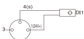
PNP型输入
