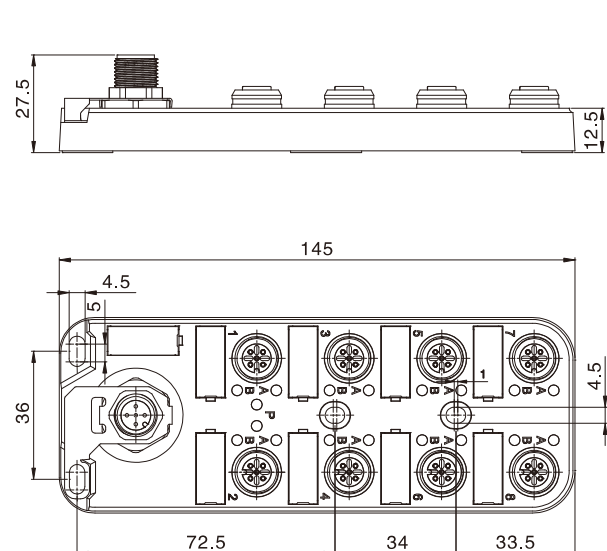
IO-Link输入输出模块-M12
