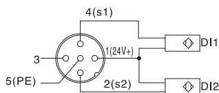
PNP型双输入
