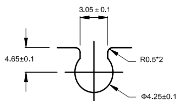
沟槽尺寸图
